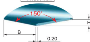
A部分詳細図
